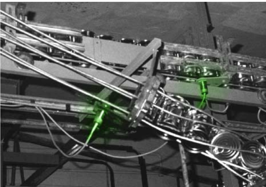
SENSORI INDUTTIVI TOTALMENTE SCHERMATI PER RILEVARE UN INTASAMENTO SUL NASTRO TRASPORTATORE.
